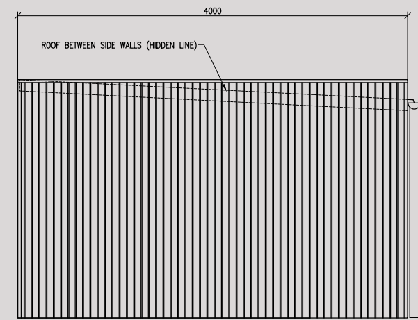
Right Elevation
