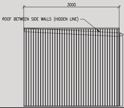
Right Elevation
