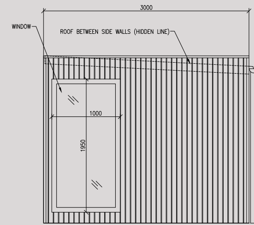
Right Elevation
