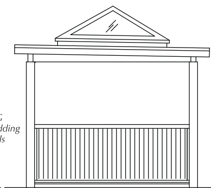
RIGHT ELEVATION
